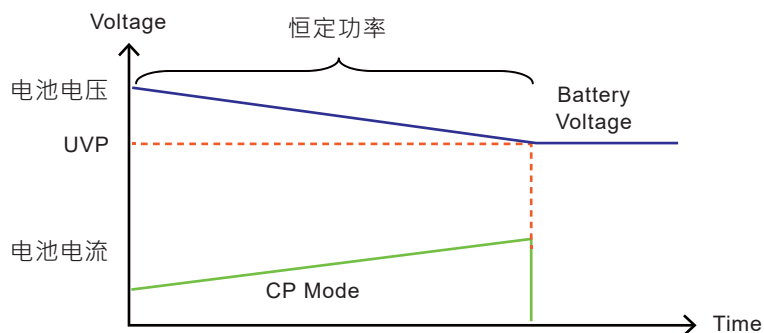
图 7：CP + UVP 电池放电测试
