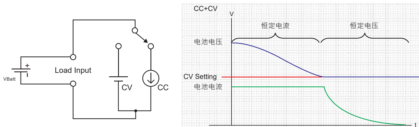
图 4：CC + CV 操作模式之应用
