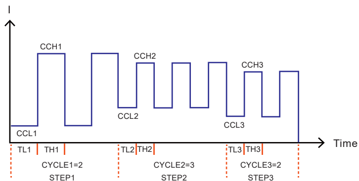
图 9：脉冲放电电流电池放电测试
