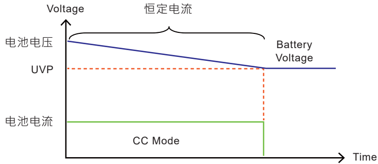
图 6：CC + UVP 电池放电测试
