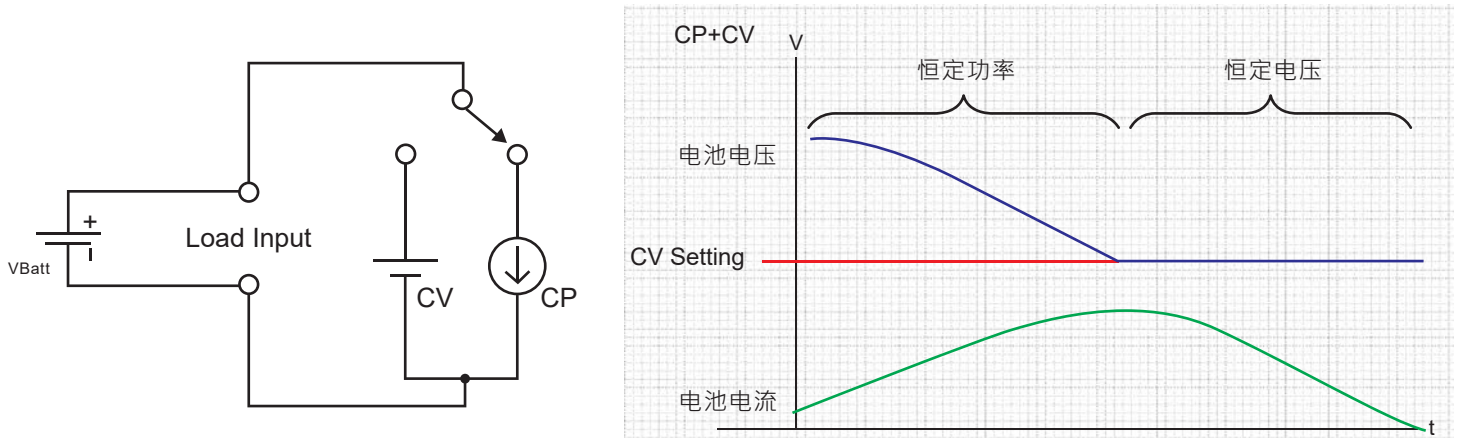
图5：CP + CV 操作模式之应用
