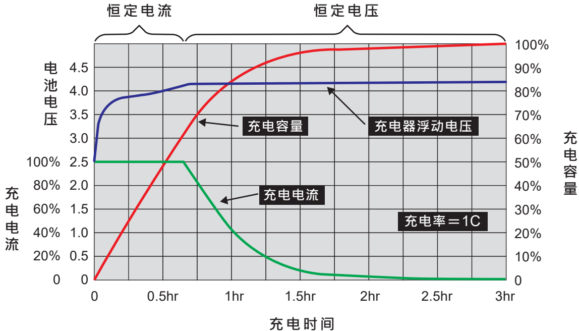
图1：显示了电池电流、电压和容量的典型充电曲线。
