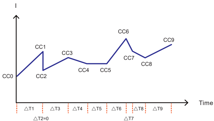
图 10：斜波模式电池放电测试
