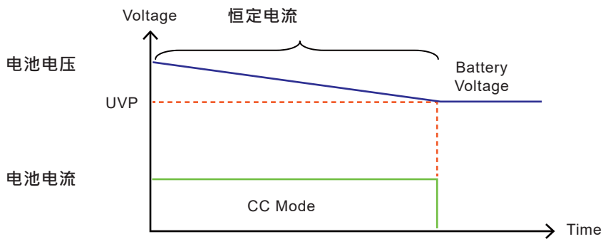
图 6 : CC + UVP 电池放电测试
