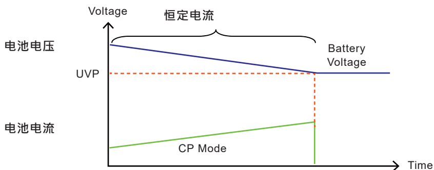
图 7 : CP + UVP 电池放电测试
