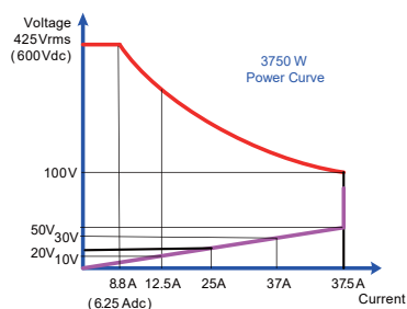
32037-425-37.5 功率曲线图
