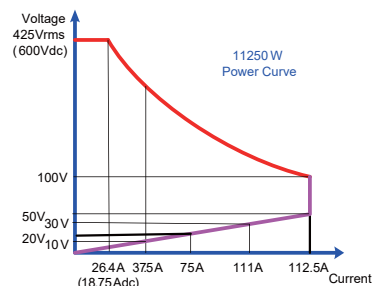
32112-425-112.5 功率曲线图
