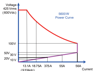
32056-425-56 功率曲线图
